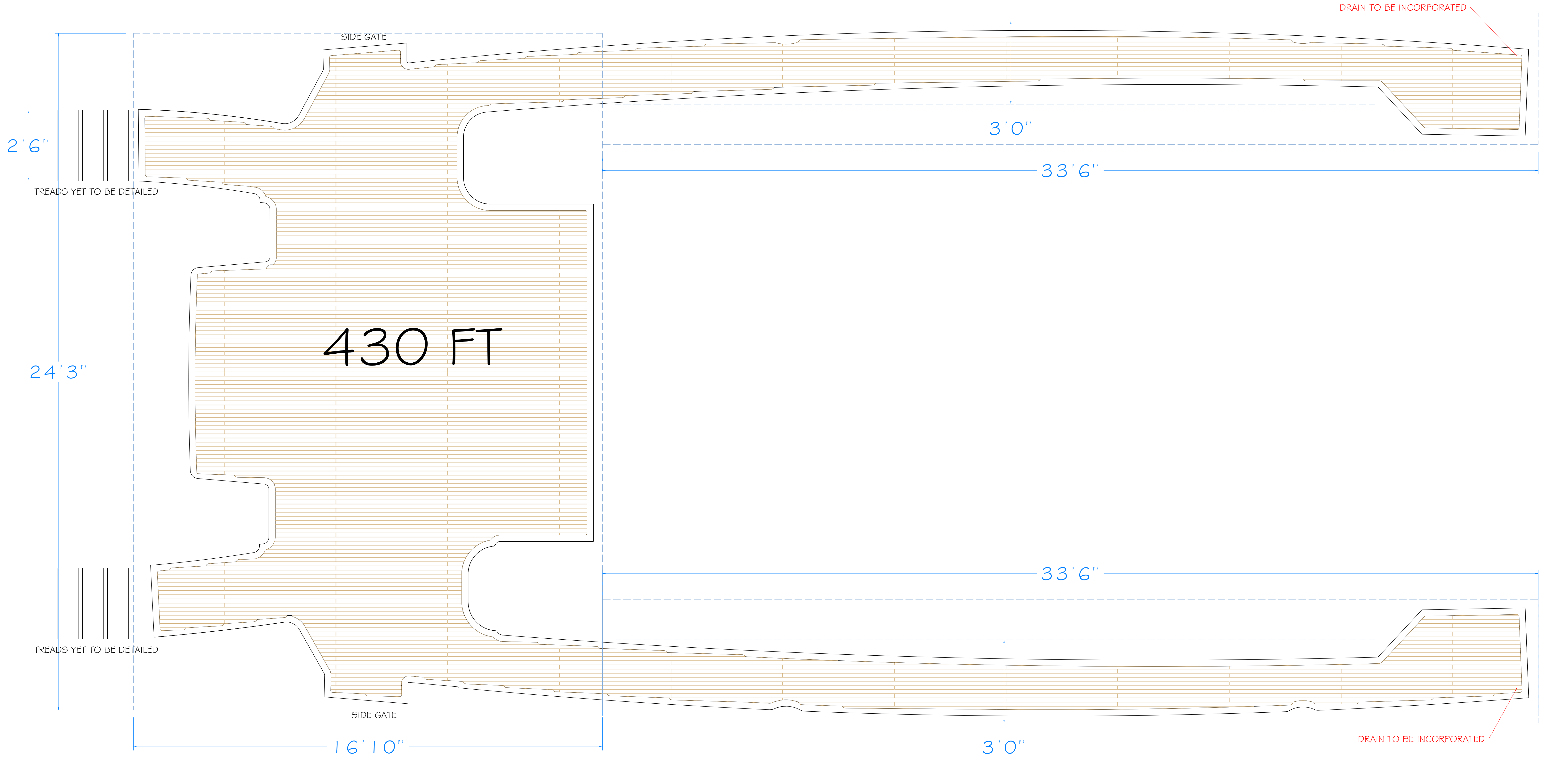
O3-MAIN DECK PLAN Scale: 1:20
