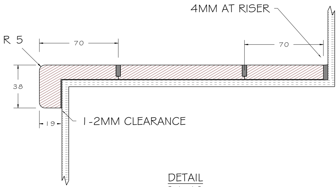
DETAIL Scale: 1:2
