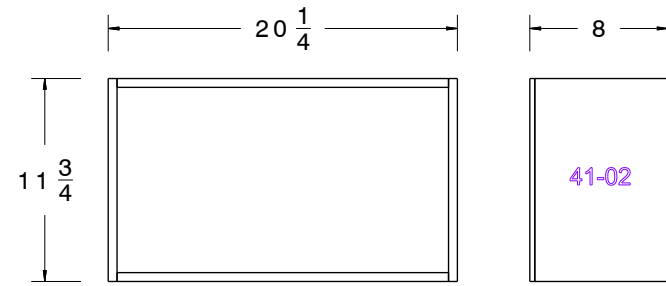
41 Scale: 1:10
