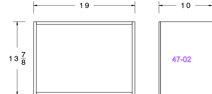
47 Scale: 1:10
