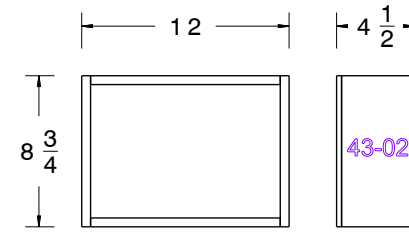
43 Scale: 1:10
