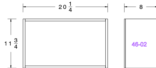
46 Scale: 1:10
