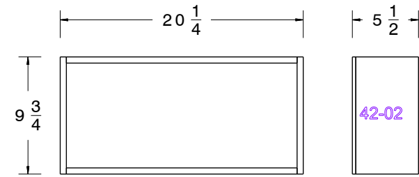
42 Scale: 1:10
