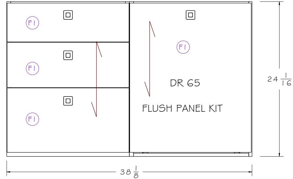
LOOKING AFT Scale: 1:8
