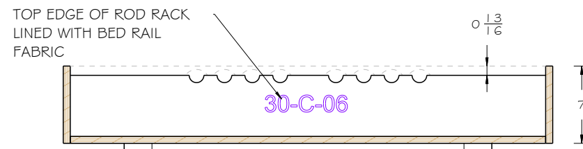
Section view G-G Scale: 1:12
