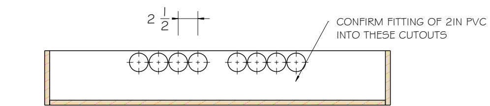
Section view G-G Scale: 1:12
